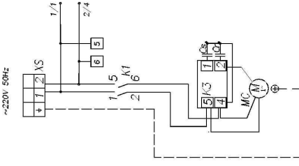
Рис.2 Питание однофазное, оставшее см.рис.1 "питание трехфазное"
