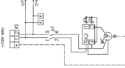
Рис.2 Питание однофазное, остальное см.рис.1 "питание трехфазное"
