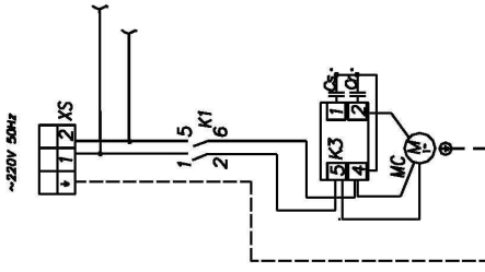
Рис.2. (однофазное питание) остальное см. рис.1
