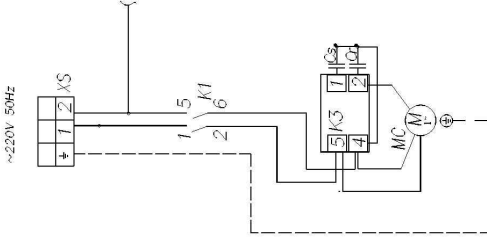
Рис. 2. (однофазное питание) остальное см. рис. 1
