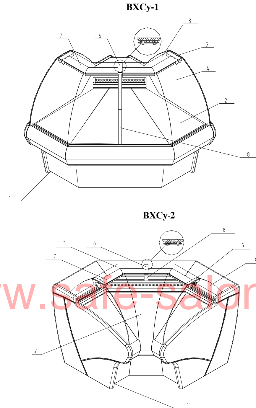
Рис.5. Схема сборки витрины.
