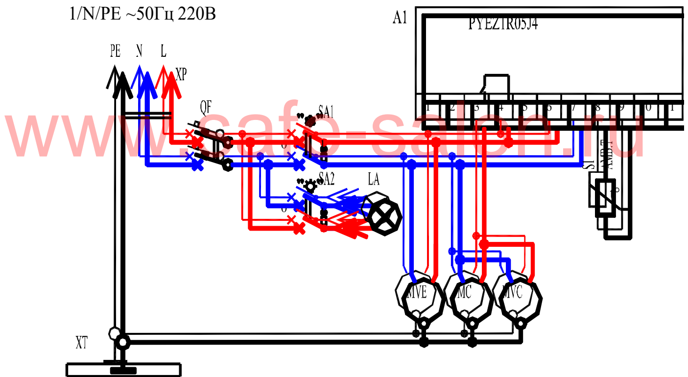
Рис.1. Схема электрическая принципиальная витрины холодильной ВХСу-1ш(2ш) Carboma.
